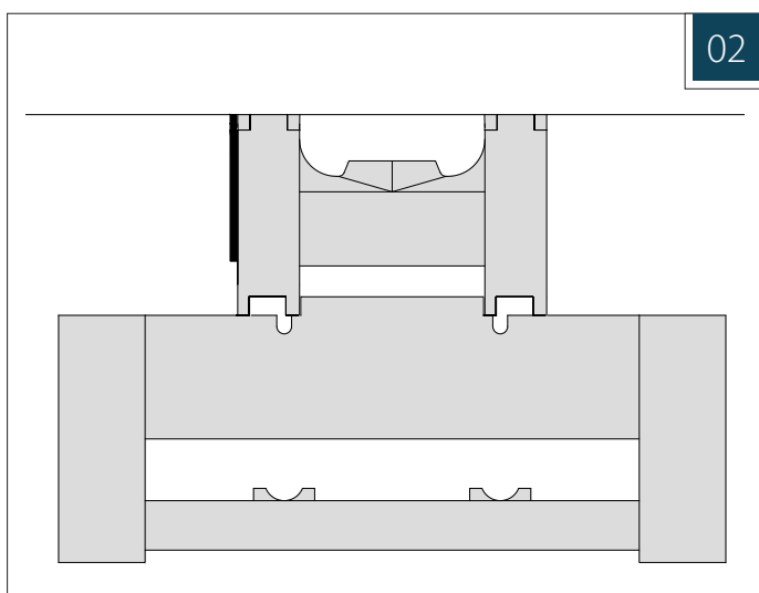
Fig. 02: Ved bruk av såleblokk, må denne bredden økes. Komprimer og avrett.
