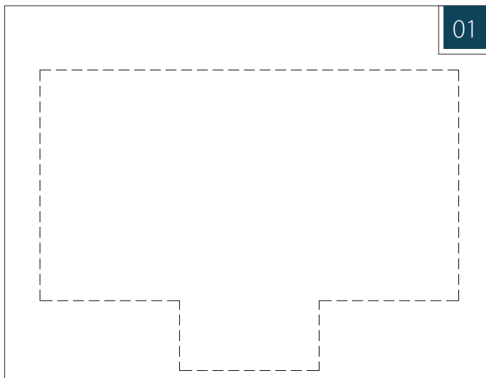
Fig. 01: Legg ut en "gate" av pukk i en bredde på ca. 50-60 cm. Marker ut hjørnene og strekk eventuelt snor.
