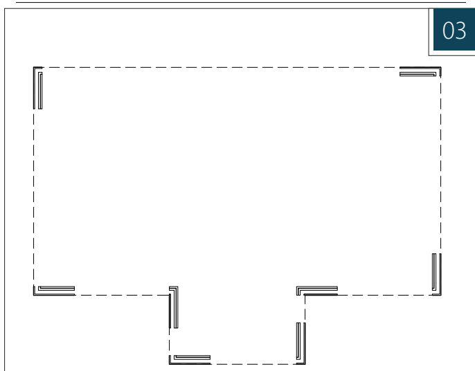
Fig. 03: Plasser ut alle utvendige og innvendige hjørneelementer med full lengde. Ved lave temperaturer kan elementene være krumme. Krummingen utløses ved å snitte innervangen fra topp til bunn i 1/4-punktene og eventuelt presse/låse elementene med trekiler.
